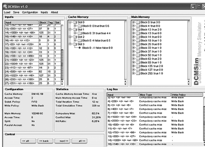
Fig. 1. Interface geral do DCMSim v1.0 .
